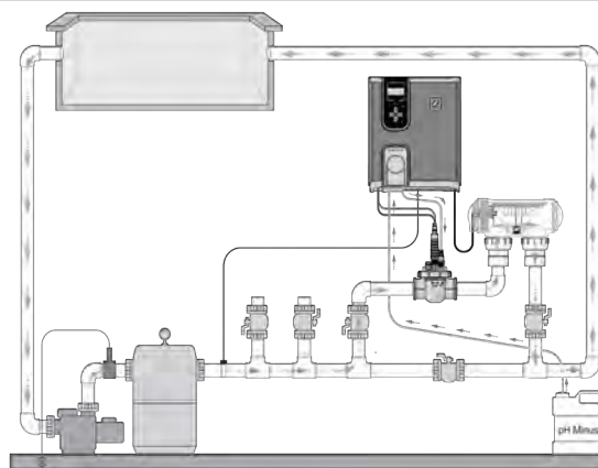
Instalación del clorador salino + módulo opcional
