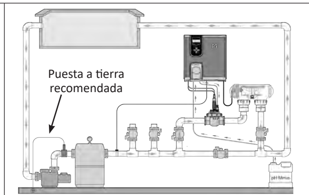
Instalación en by-pass
